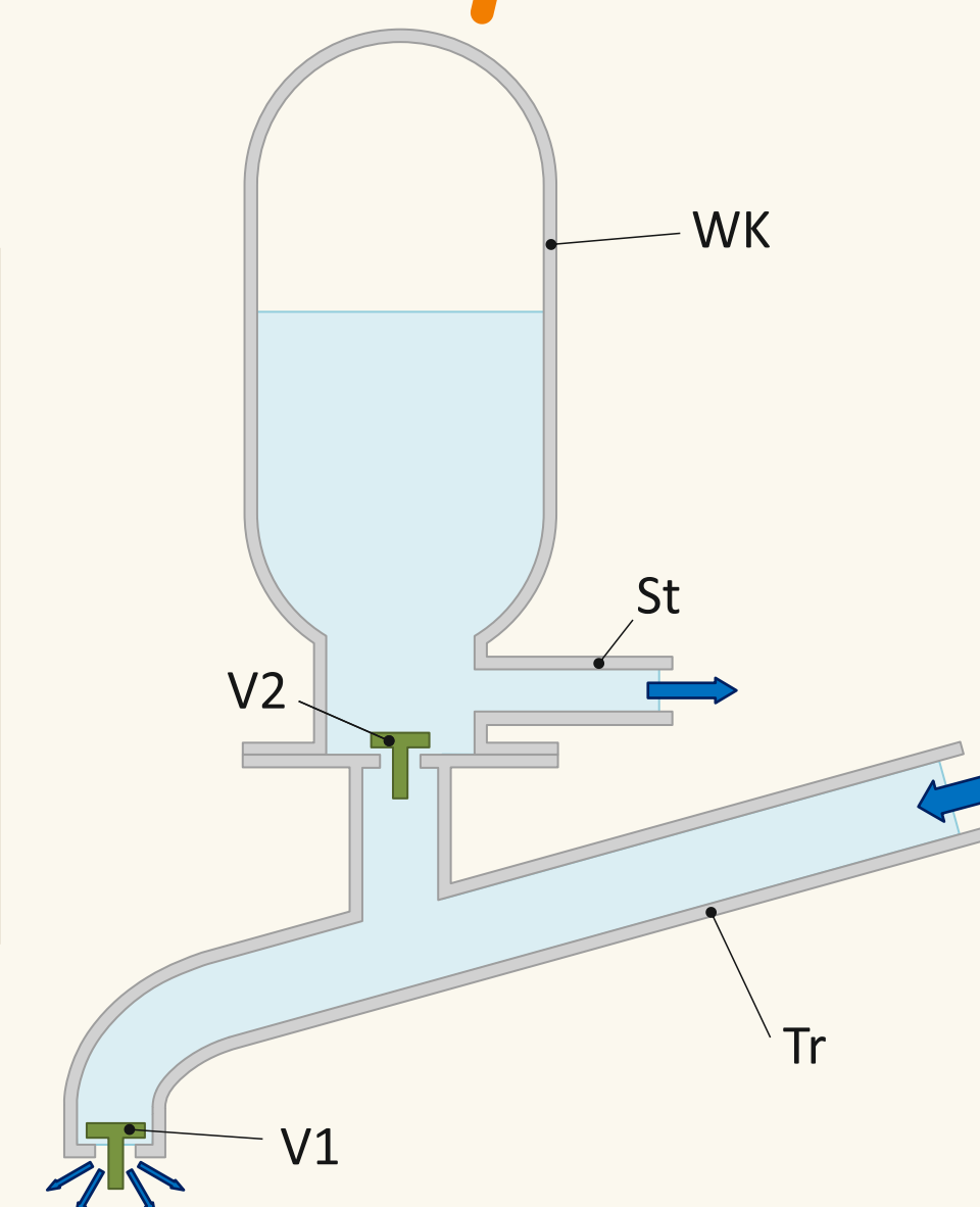
Hauptbauteile des hydraulischen Widders Windkessel [WK], Stoßventil [V1], Druckventil [V2], Steigleitung [St], Triebleitung [Tr]
